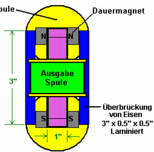
QUERSCHNITT A-A
