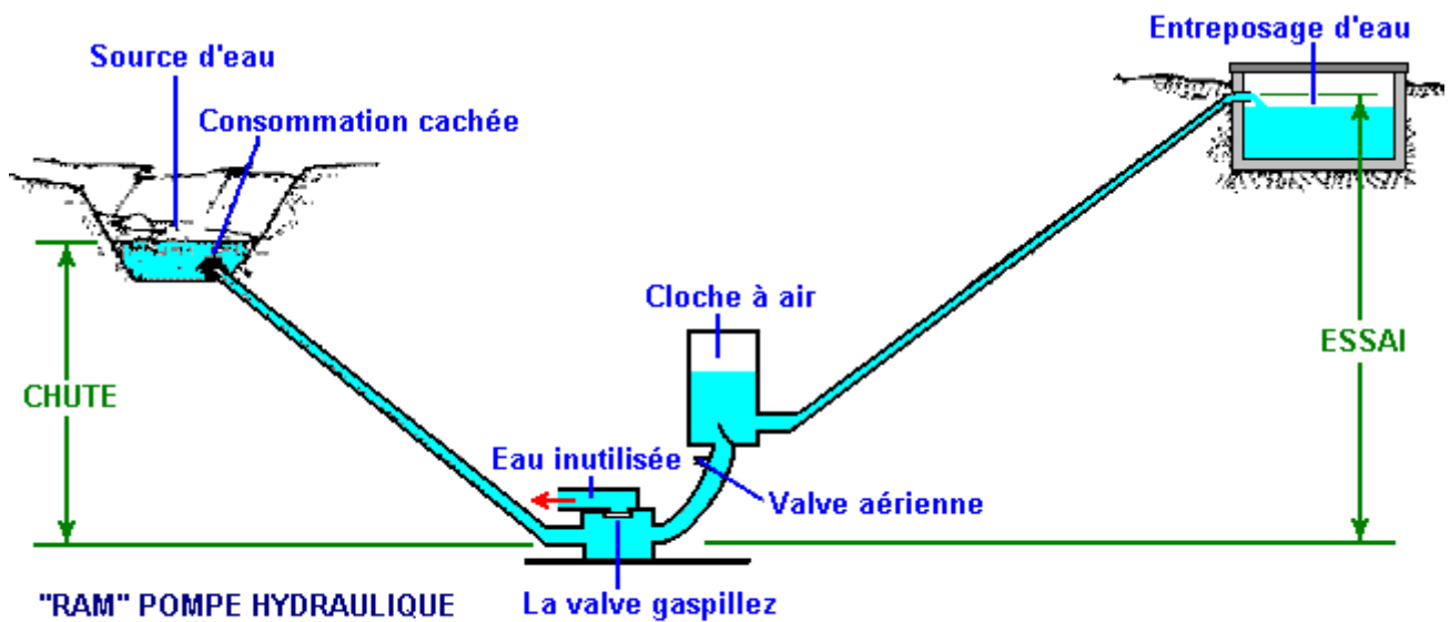
Diagramme de : www.thefarm.org/charities/i4at/lib2/hydrpump.htm
