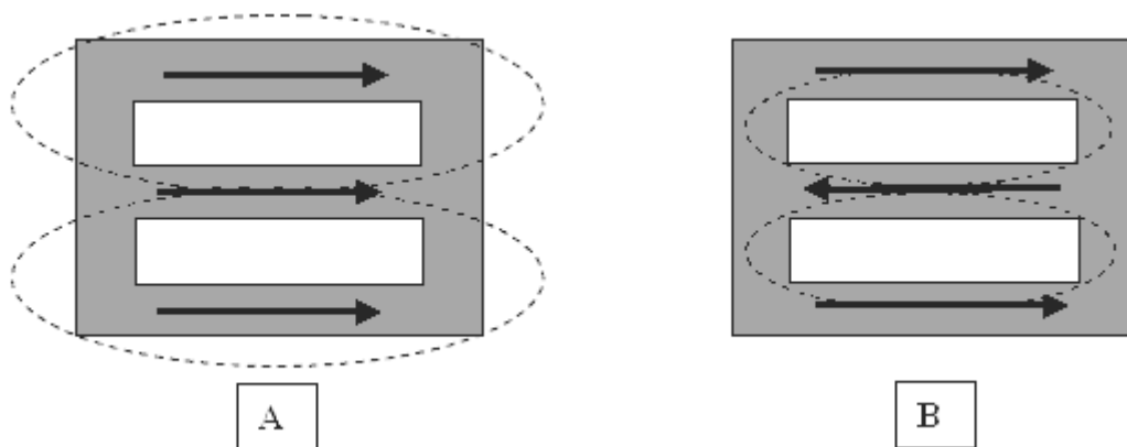
Fig. 12. La direzione del campo magnetico all'interno il ferromagnetico nucleo per la magnetizzazione - (A) e smagnetizzazione - (B).
