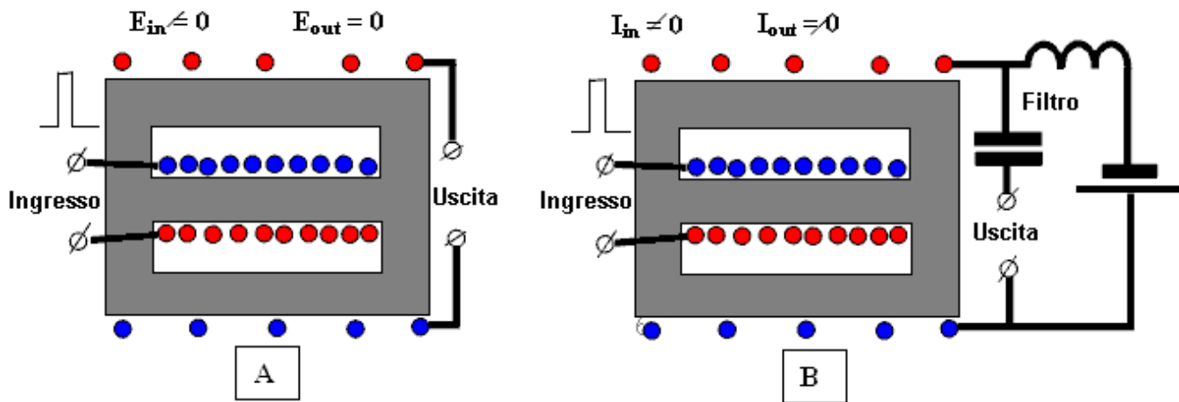
Fig. 11. Un semplice "smagnetizzazione" schematica basata su nuclei a forma di E.
